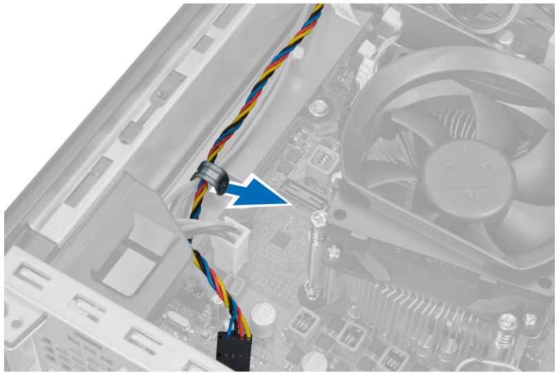
5. שחרר את כבלי מאוורר המערכת מהתפס שבמארז.
