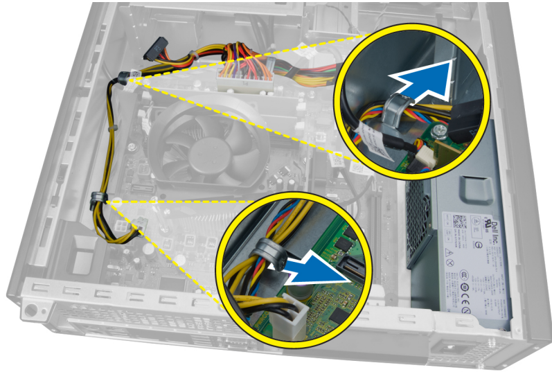
5. לחץ על הכבל בעל 24 הפינים והרם אותו כדי לנתקו מלוח המערכת.
