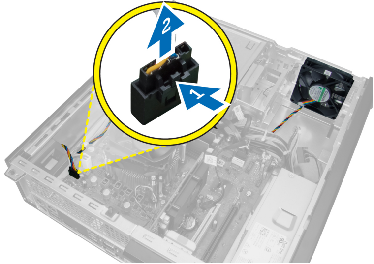
4. שלוף את כבל מאוורר המערכת מהתפס שבמארז.
