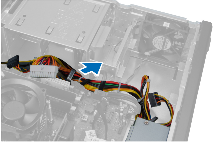
7. שלוף את כבלי ספק הכוח מהתפס שבמארו.
