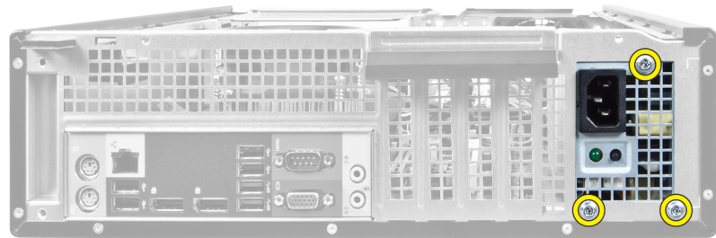
9. לחץ על לשונית השחרור הכחולה שלצד ספק הכוח והחלק את ספק הכוח לכיוון חזית המחשב.
